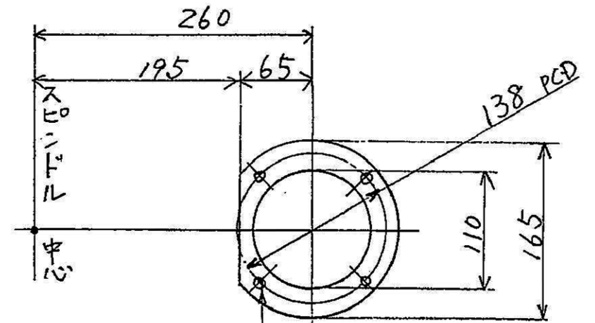
4-φ14 (等配) A 矢視 (コラムフランジ取付部)
