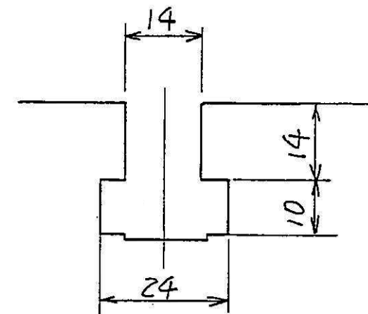
T溝寸法
