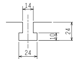
T溝詳細図
